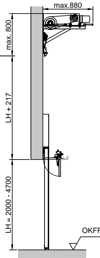
Vertikalschnitt
