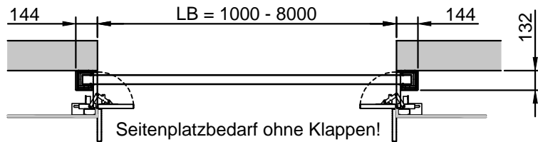
Horizontalschnitt
