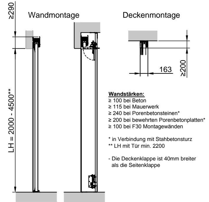
Seitenklappe "optional"
