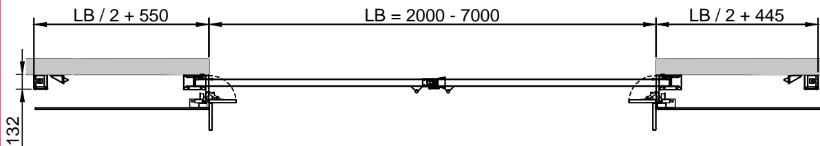
Horizontalschnitt
