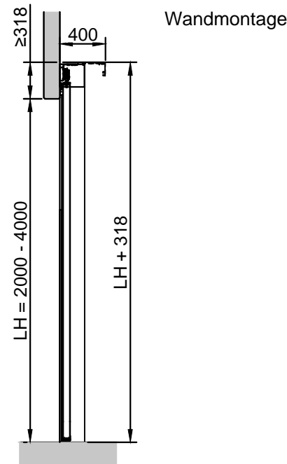
Vertikalschnitt
