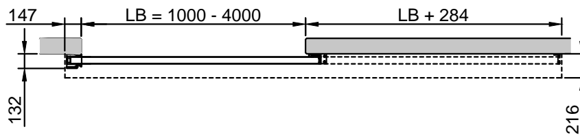
Horizontalschnitt
