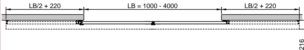
Horizontalschnitt
