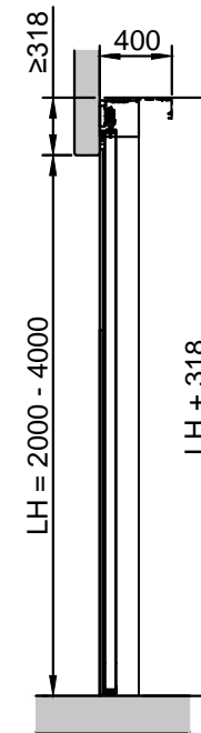
Vertikalschnitt
