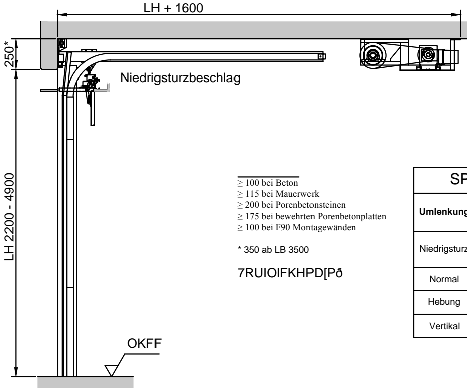
Vertikalschnitt
