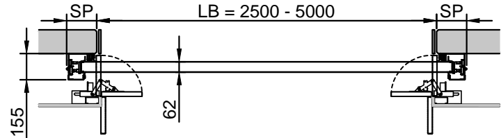
Horizontalschnitt
