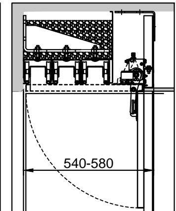
Deckenklappe "optional"
