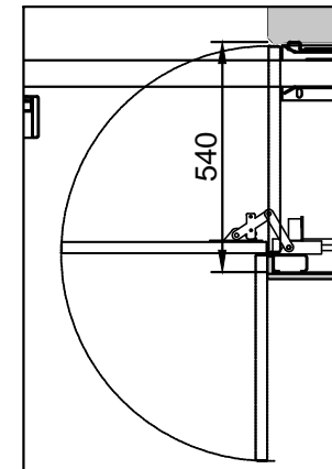
Seitenklappe "optional"
