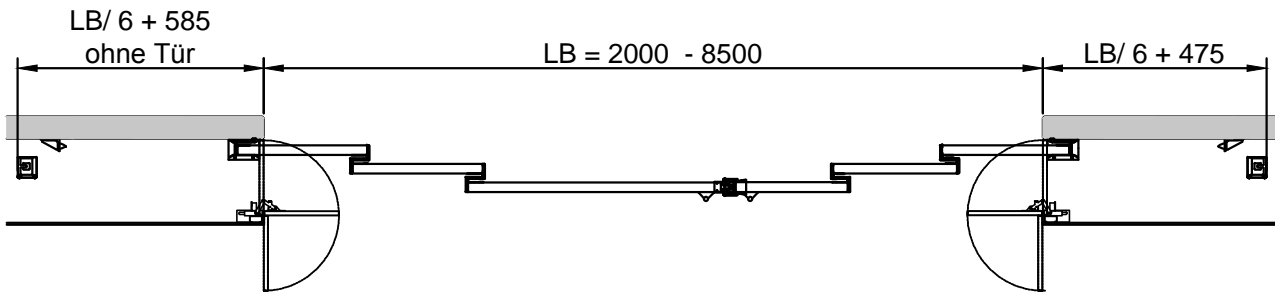
Horizontalschnitt
